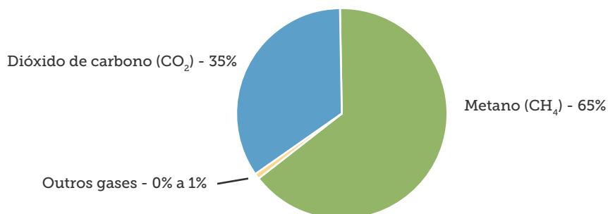
Composição média do biogás
