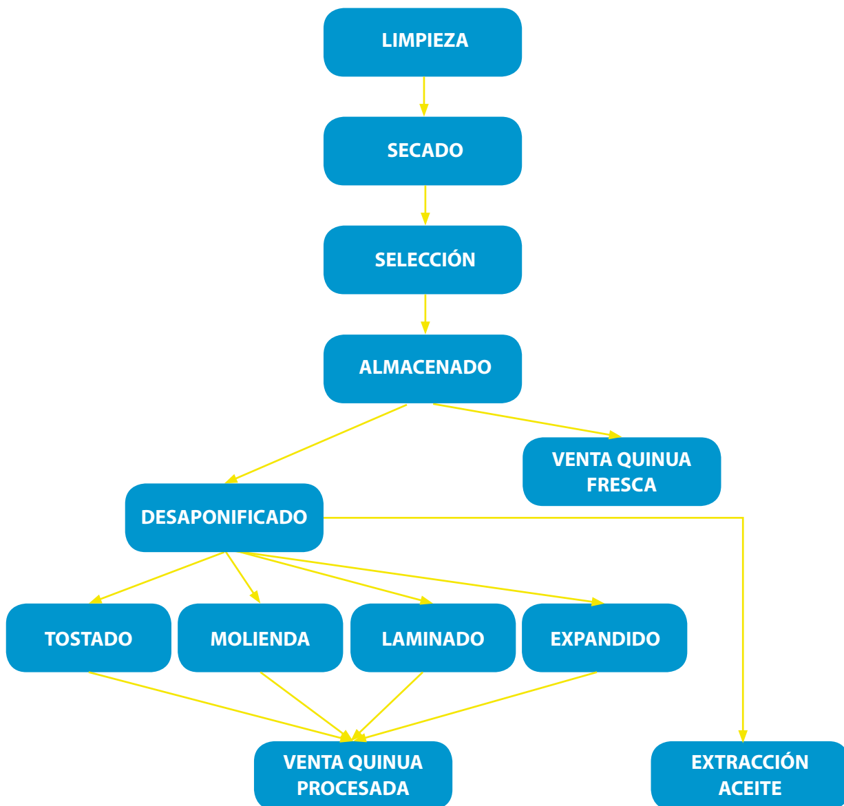
Figura 1. Flujograma de procesamiento de quinua.
