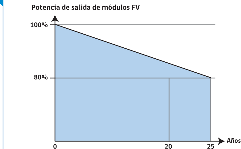
Ilustración 2 Gráfico de potencia de salida de módulos FV con relación a potencia nominal (Fuente: Elaboración propia)
