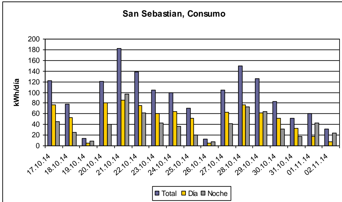
Ilustración 6: Consumo medido
