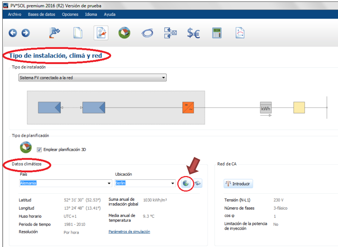
Ilustración 10 – Tipo de instalación, clima y red en PVSol
