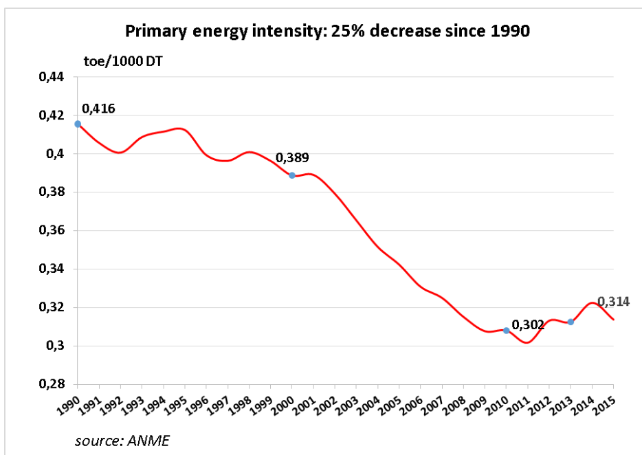
Figure 13: Evolution de l'intensité d'énergie primaire en Tunisie
