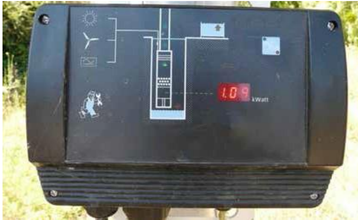
Controlador con visualizador e indicador LED de fallo
