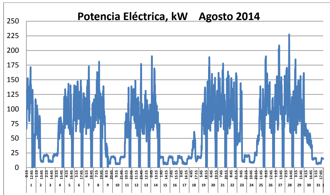
Figura N° 3-5: Perfil de Demanda de Potencia del Mes de Agosto 2014
