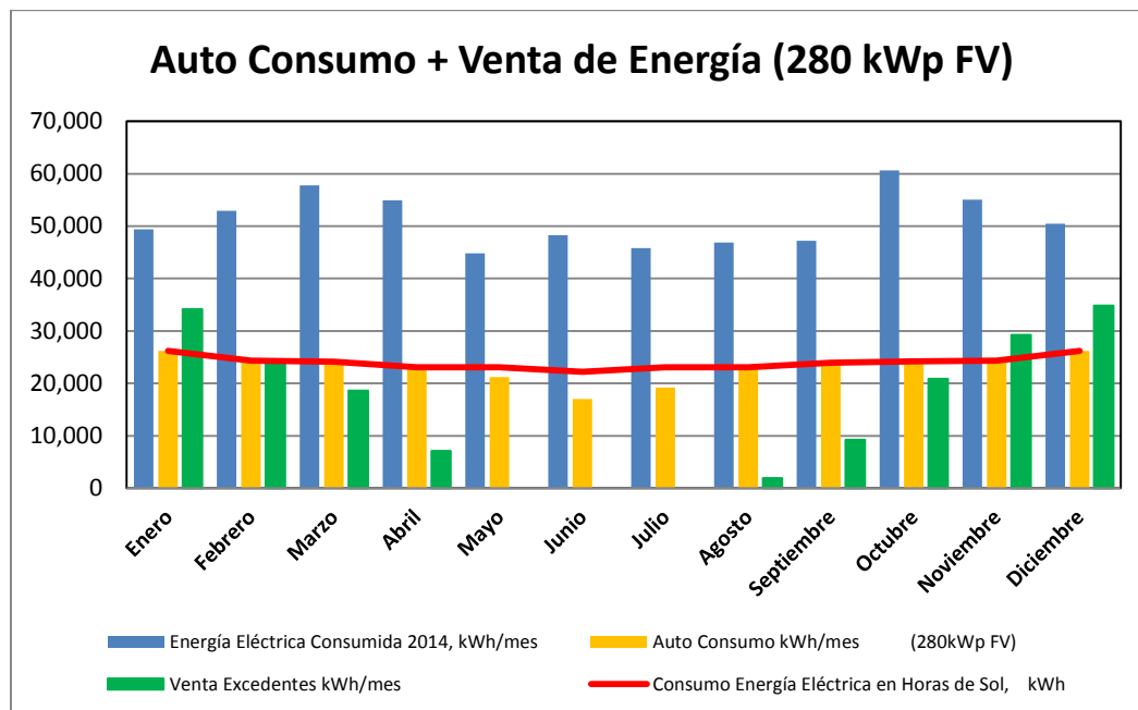
Figura N° 3-8: Distribución de autoconsumo y venta de energía en año 1
