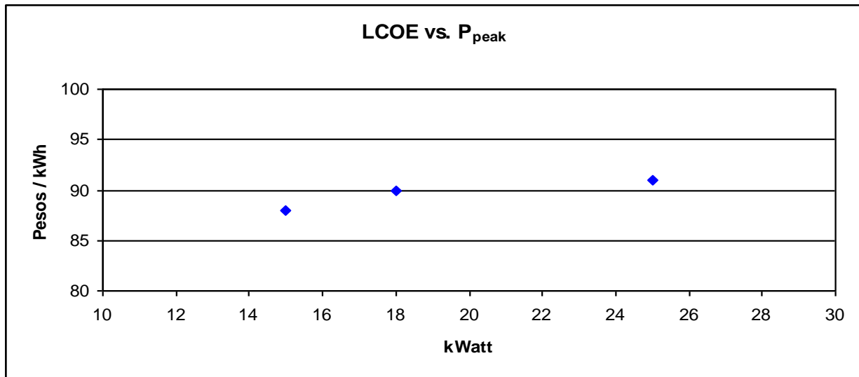
Ilustración 21: LCOE versus diferentes tamaños del sistema solar
