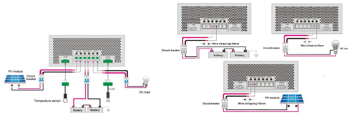
Spajanje invertora sa odgovarajućim komponentama
