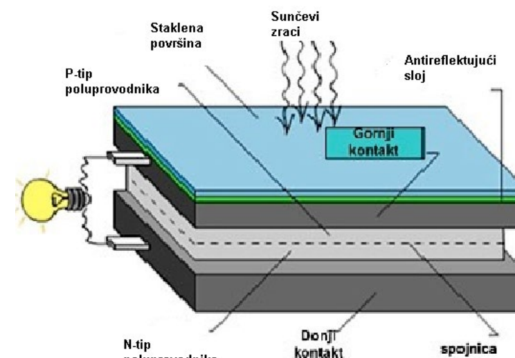
Fotonaponska ćelija
