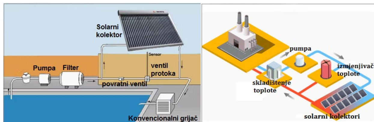
Šematski prikaz upotrebe kolektora za grijanje vode u bazenu
