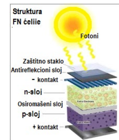
Struktura FN ćelije
