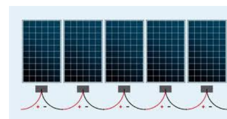
Serijsko vezivanje panela
