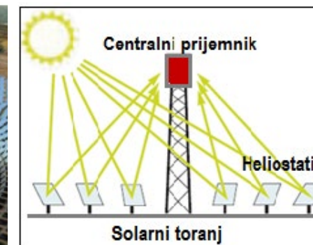
Šematski prikaz solarnog tornja
