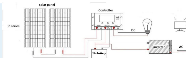
Šematski prikaz serijskog vezivanja panela
