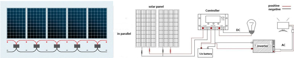
Paralelno vezivanje panela
