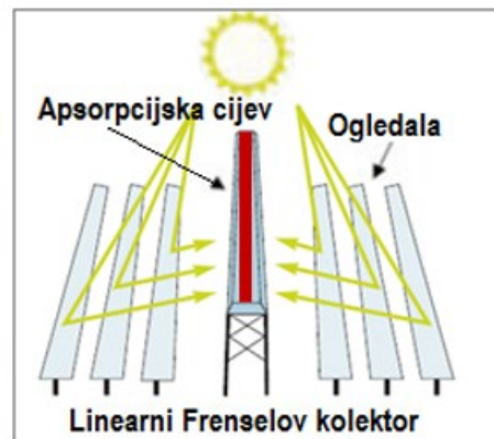
Linearni Fresnelovi kolektori kolektori - šematski prikaz
