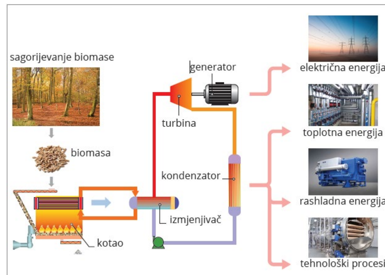
Šematski prikaz ORC sistema na biomasu
