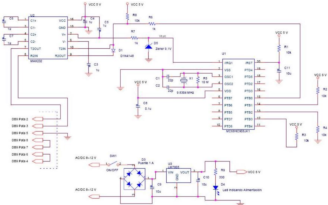
Figura 5. Diagrama esquemático del circuito programador
