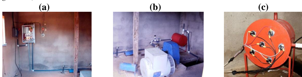
Figura 10. a), b) Regulador electrónico instalado en una MCH de Nicaragua c) Banco disipador de potencia del sistema
