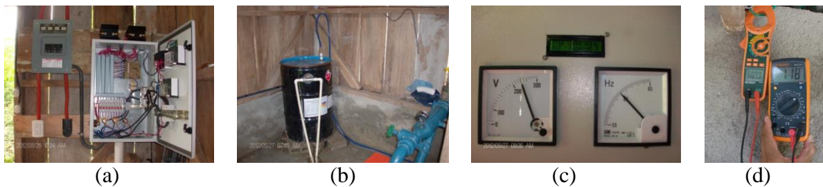
Figura 9. a) Gabinete de regulación instalado. b) Banco disipador de potencia instalado. c) Sistema en Funcionamiento d) Medición residencial del servicio eléctrico.
