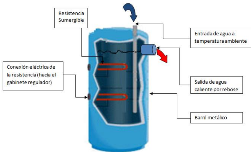
Figura 6. Esquema de funcionamiento del banco disipador de potencia.
