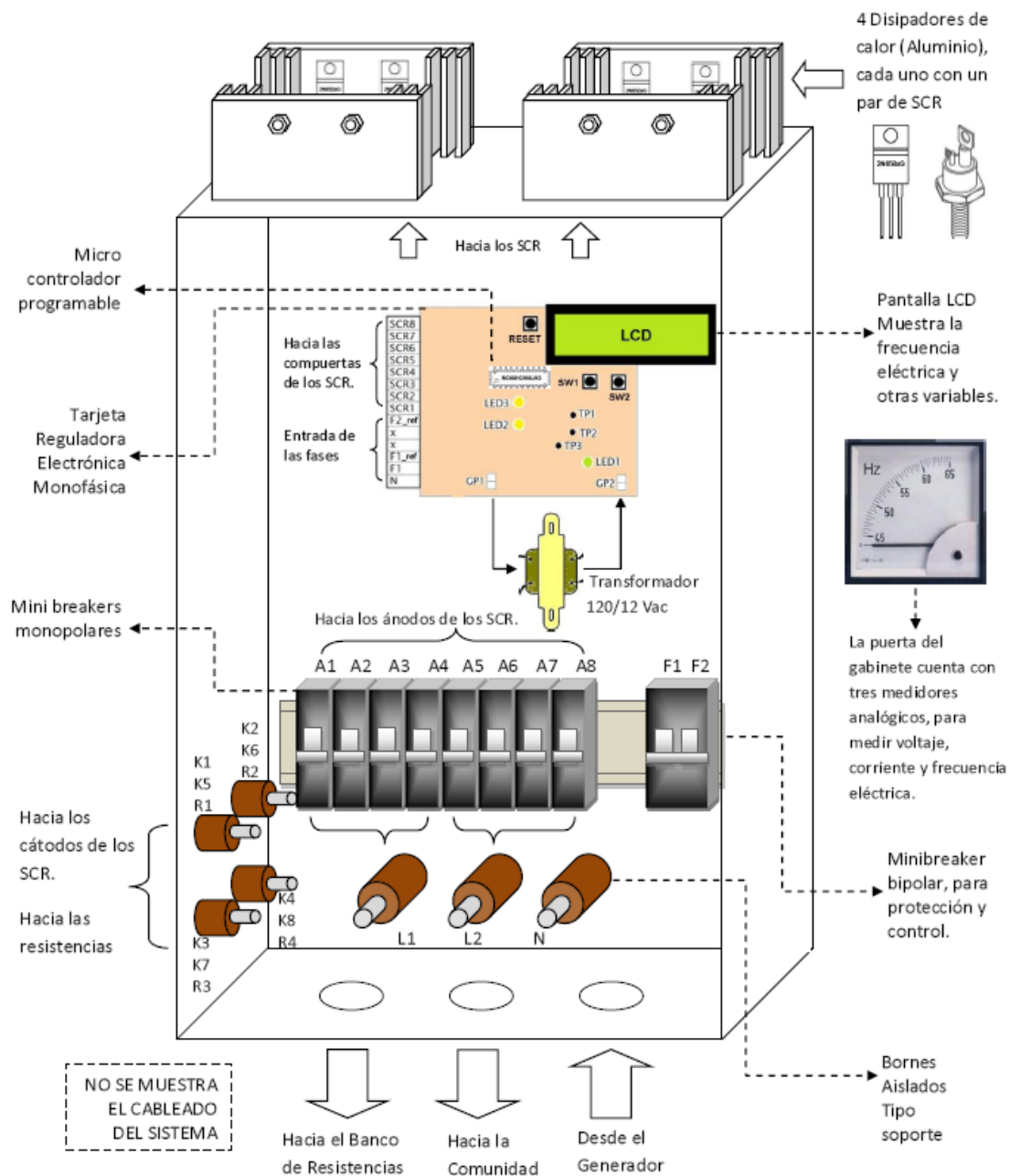
Figura 2. Diagrama pictórico con los elementos del gabinete regulador electrónico
