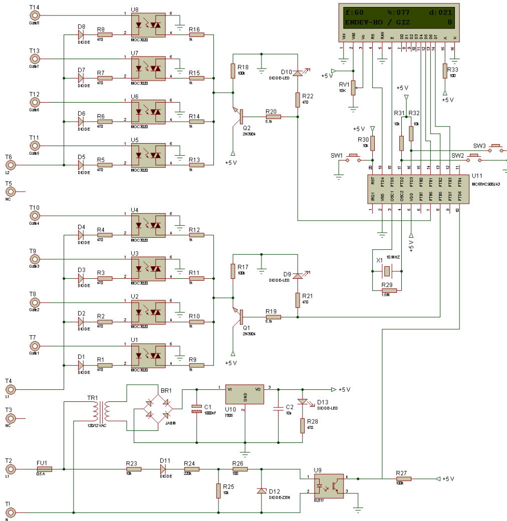
Figura 3. Diagrama esquemático la tarjeta electrónica monofásica.
