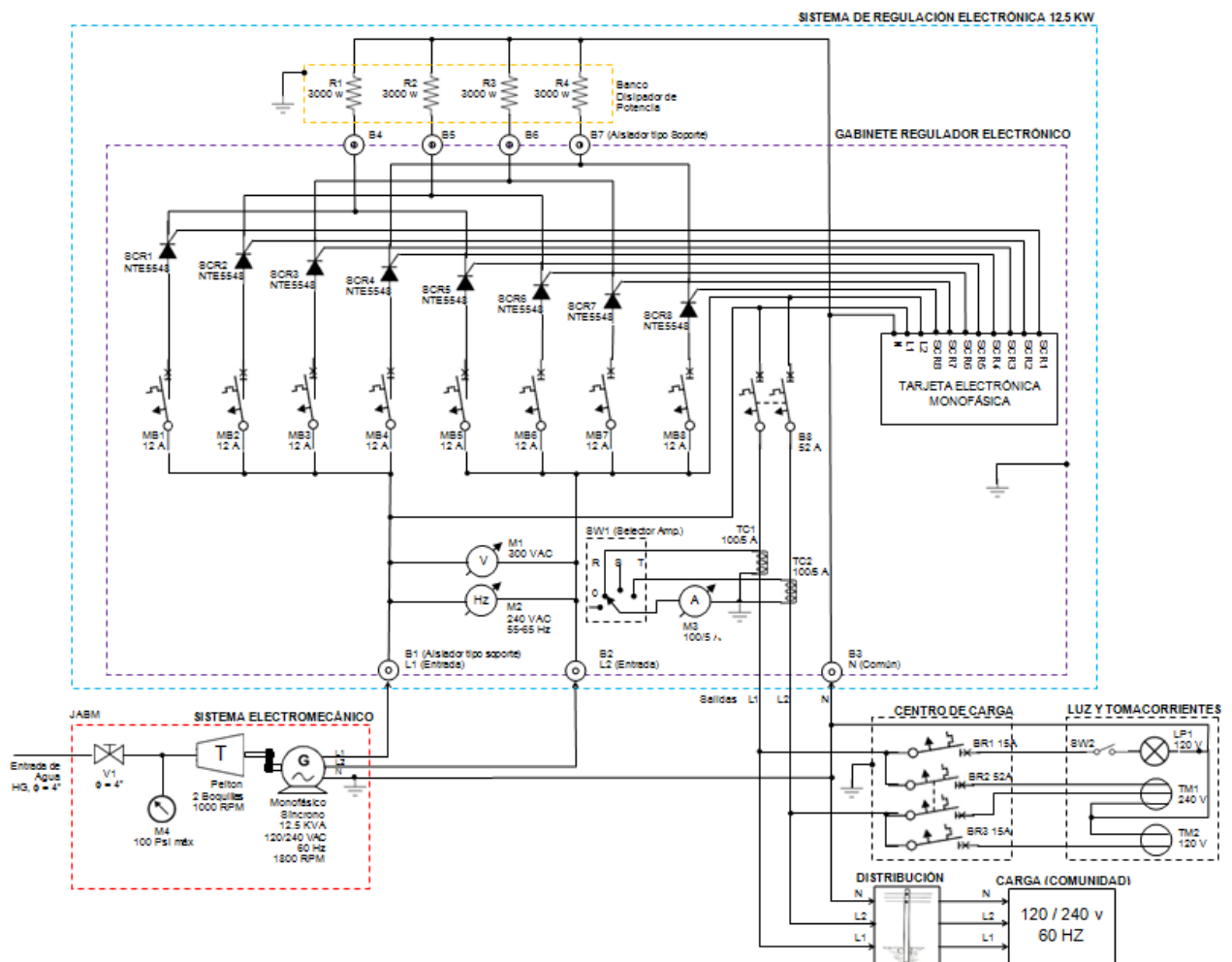
Figura 1. Diagrama esquemático de una pequeña MCH con Sistema Regulador Electrónico de Carga
