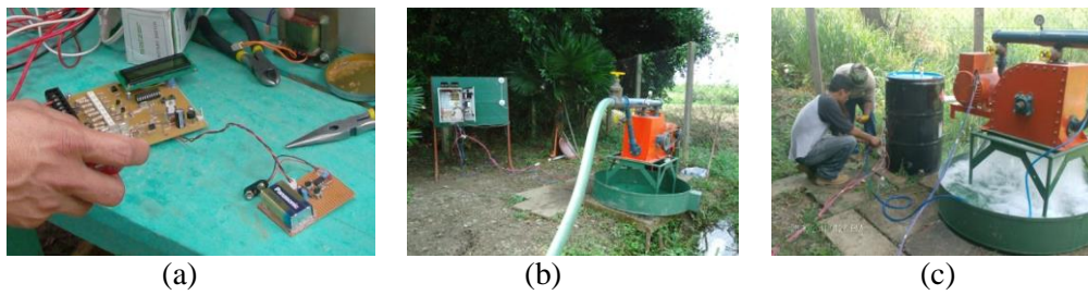
Figura 8. a) Pruebas con circuito generador de frecuencias. b), c) Pruebas con generador eléctrico, turbina y bomba de agua.
