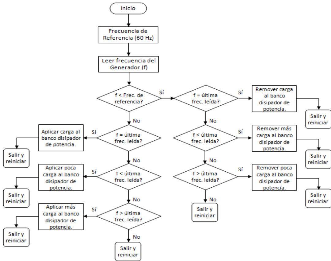
Figura 4. Diagrama de flujo del proceso de regulación de frecuencia.
