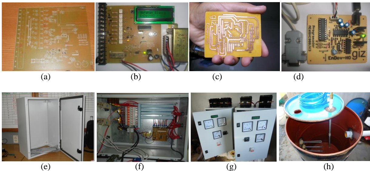
Figura 7. a), b) Tarjeta electrónica. c), d) Circuito programador. e), f), g) Gabinete regulador. h) Banco disipador de potencia.
