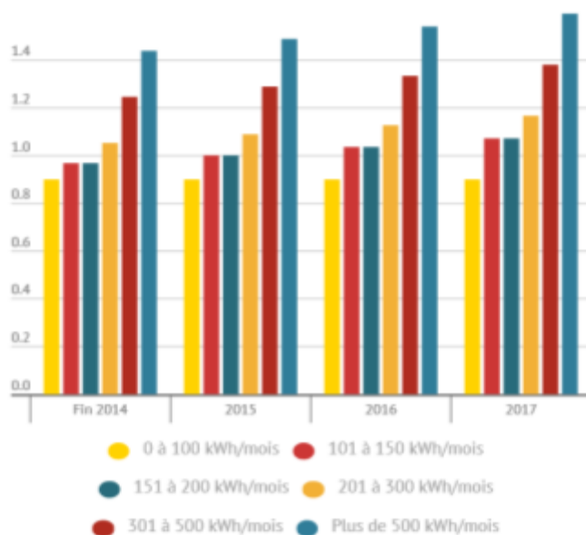
Figure 4 : Évolution du prix de l'électricité en basse tension (Tarifs ONEE en Dh/kWh)
