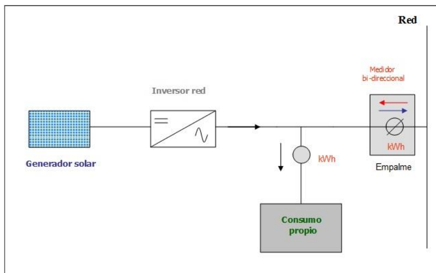
Ilustración 4: Esquema sistema fotovoltaico.
