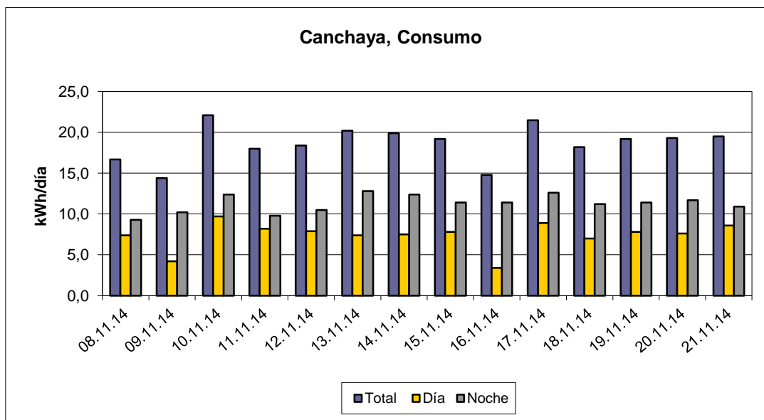
Ilustración 5: Consumo medido
